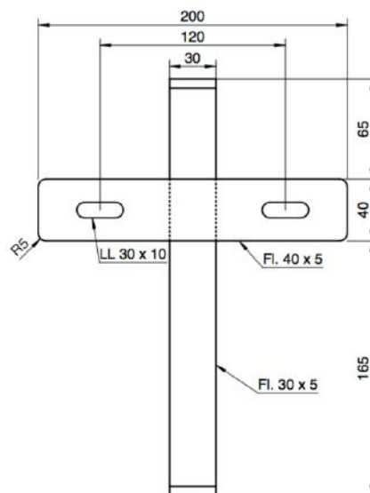
MASTHALTER VARIO-2
