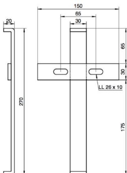
MASTHALTER VARIO-1
